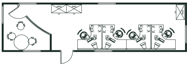
TN154 Bureaux Titan avec salle de réunion cloisonnée Surface au sol de 53.78 m 2
