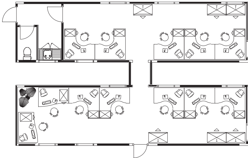
PK 402 Complexe de bureaux Pacemaker avec sanitaires - surface totale au sol 76,04 m 2
